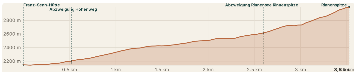
Profilo altimetrico
