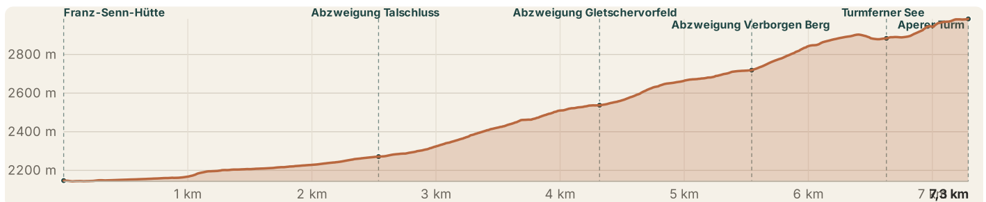
Profilo altimetrico
